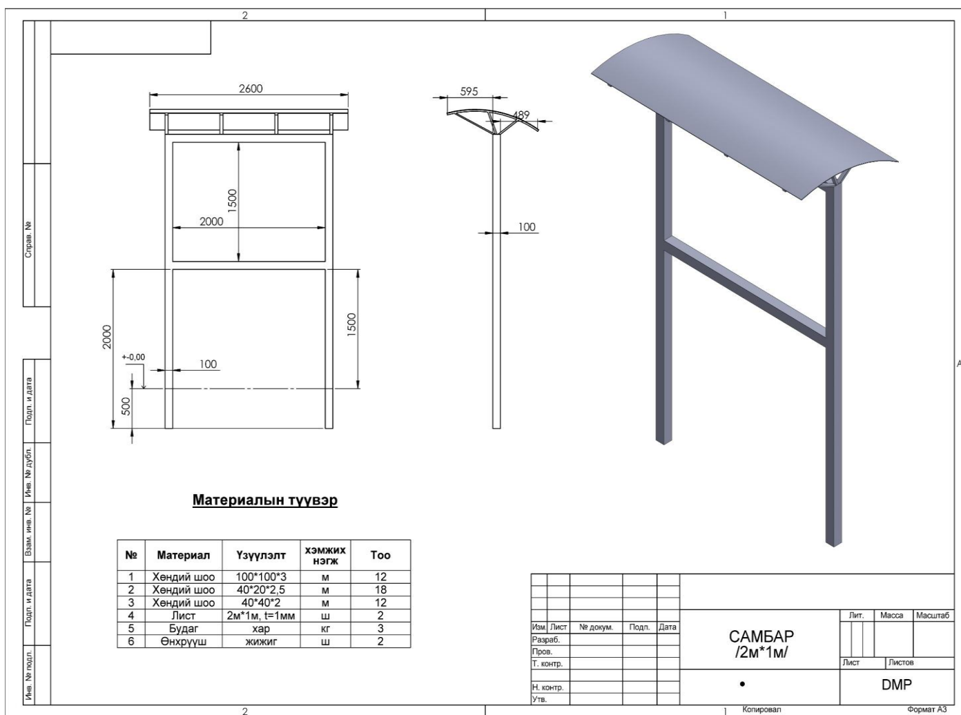
Хавсралт-1. Гэрэлтэй самбарын ажлын зураг:
