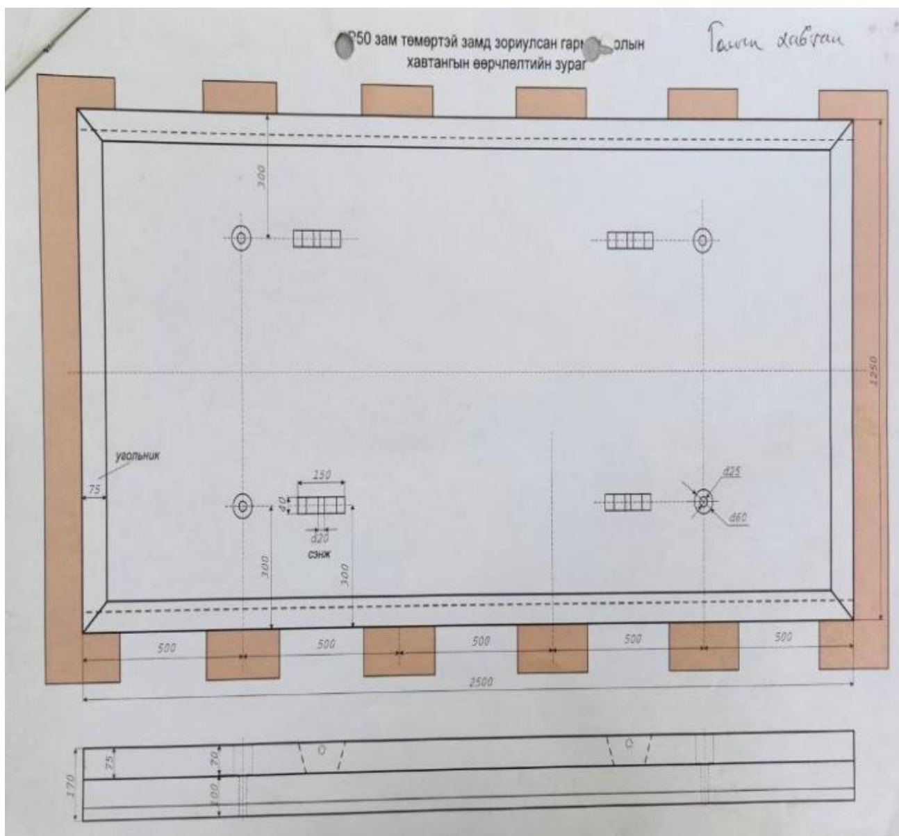
Зураг 1. Хийцлэлийн хэмжээст зураг
